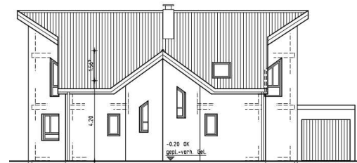
Ostansicht ( Straße )
